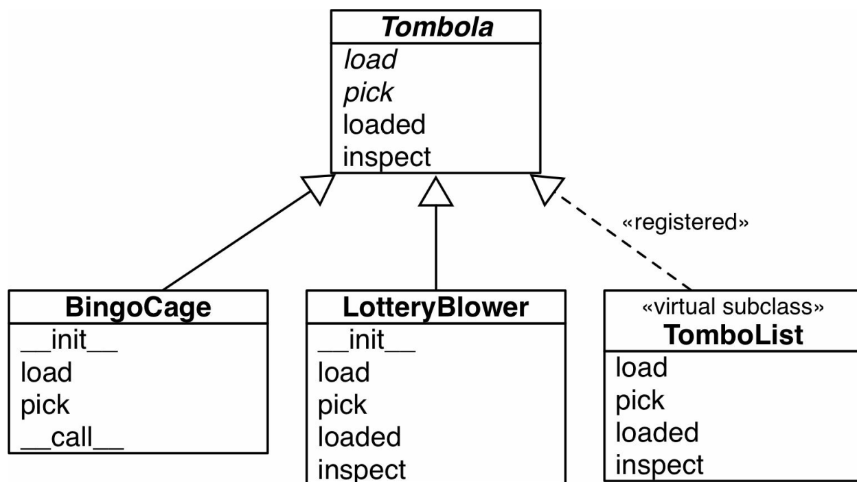
图 13-5：一个抽象基类和 3 个子类的 UML 类图。 根据 UML 的约定，抽象基类 Tombola 和它的抽象方法使用斜体。虚线箭头表示接口实现，这里表示 TomboList 不仅实现了 Tombola 接口，还被注册为 Tombola 的虚拟子类（详见本章后文） 8
