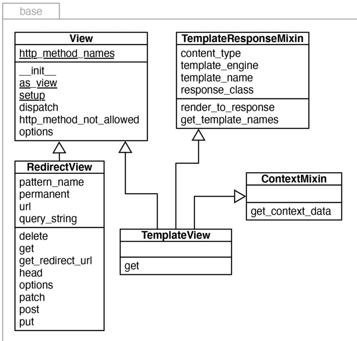
图 14-3: django.views.generic.base 模块的 UML 类图
