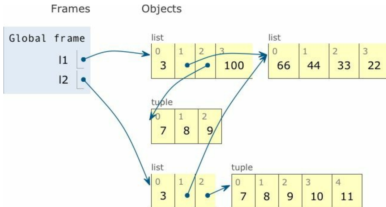
图 6-4: l1 和 l2 的最终状态：二者依然引用同一个列表对象，现在列表的值是 [66, 44, 33, 22]，不过 l2[2] += (10, 11) 操作创建一个新元组，内容是 (7, 8, 9, 10, 11)，它与 l1[2] 引用的元组 (7, 8, 9) 无关（截图由 Python Tutor 网站生成）
