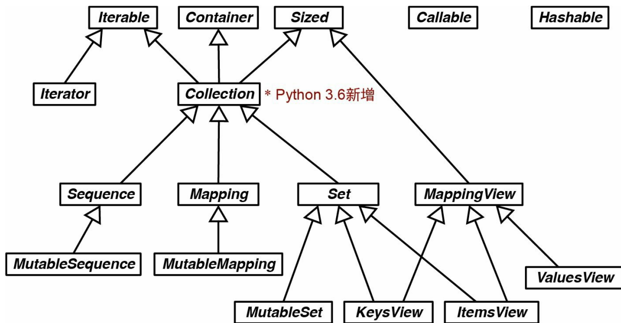
图 13-4: collections.abc 模块中抽象基类的 UML 类图
