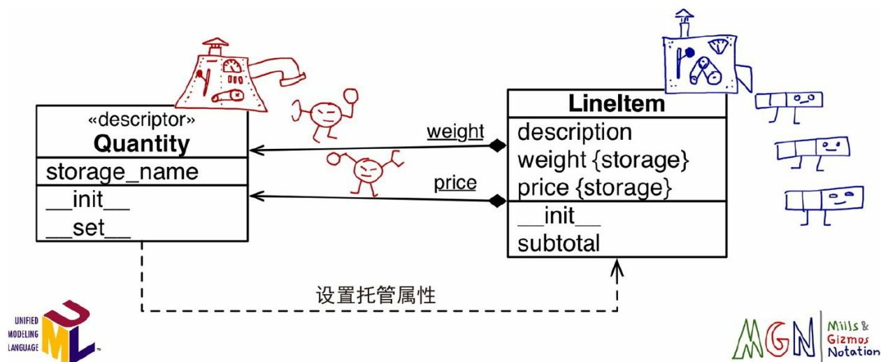
图 23-2：带有 MGN（Mills & Gizmos Notation，机器和小怪兽图例法）注解的 UML 类图：类是机器，用于生产小怪兽（实
