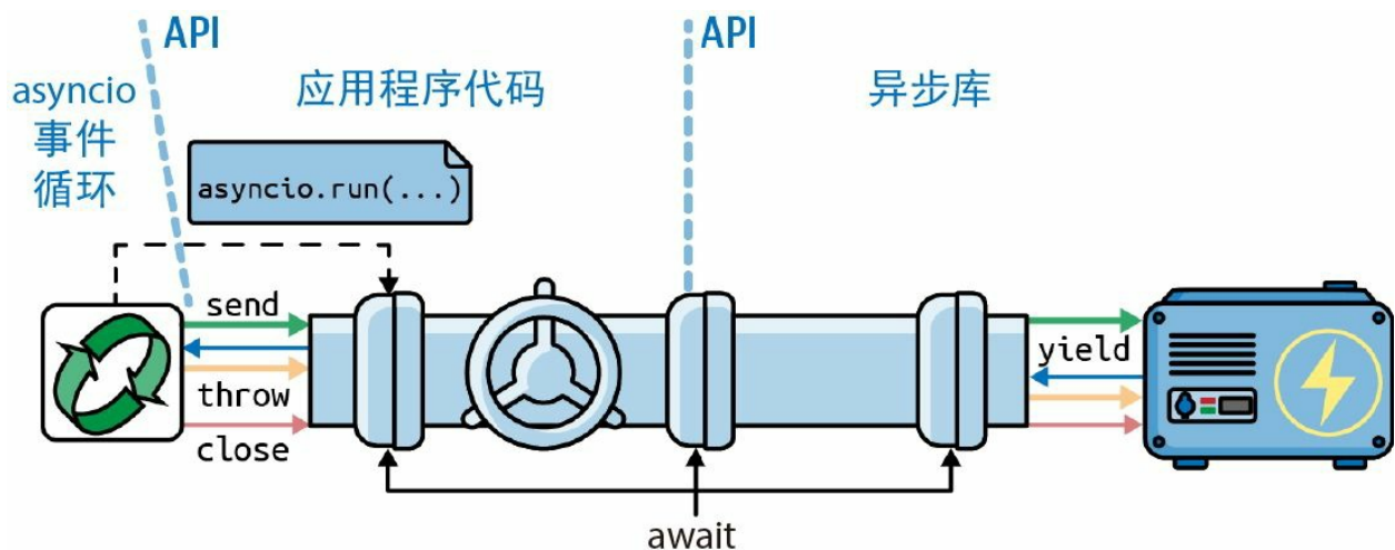
图 21-1：在异步程序中，用户编写的函数启动事件循环，使用 asyncio.run 调度最初的协程。用户编写的各个协程使用 await 表达式驱动下一步，构成一个通道，打通 HTTPX 等库与事件循环
