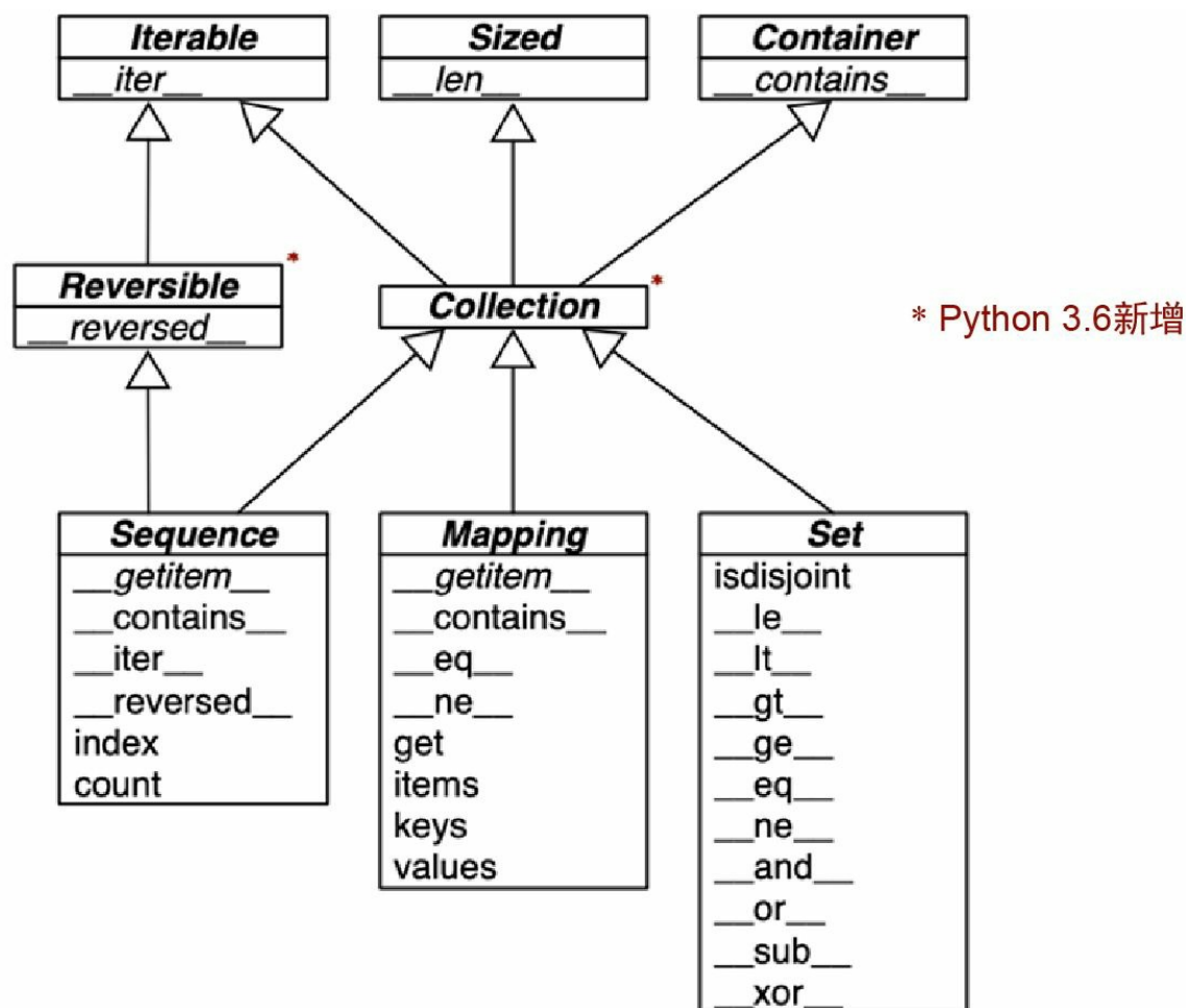
图 1-2：基本容器类型的 UML 类图。以斜体显示的方法名称表示抽象方法，必须由具体子类（例如 list 和 dict）实现。其他方法有具体实现，子类可以直接继承
