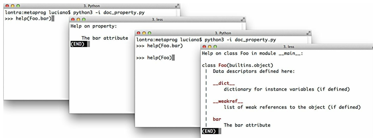
图 22-1：在 Python 控制台中执行 help(Foo.bar) 命令和 help(Foo) 命令时的截图，源码在示例 22-26 中
