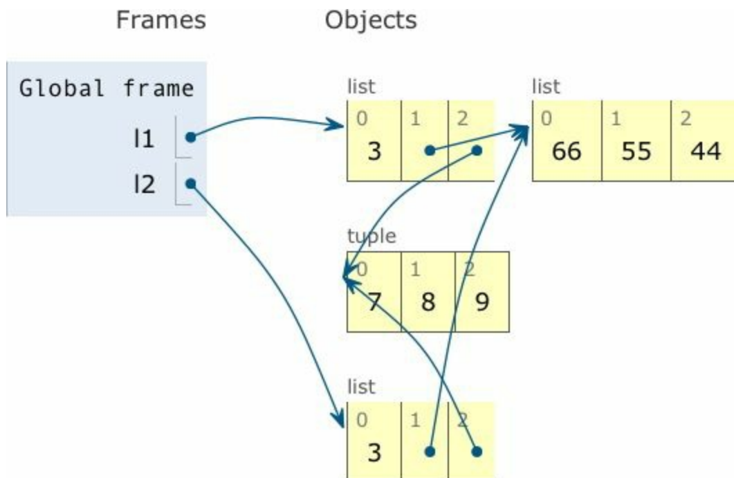
图 6-3: 示例 6-6 执行 l2 = list(l1) 赋值后的程序状态。11 和 12 引用不同的列表，但是这两个列表内的 [66, 55, 44] 列表和 (7, 8, 9) 元组引用的是相同的对象（截图由 Python Tutor 网站生成）
