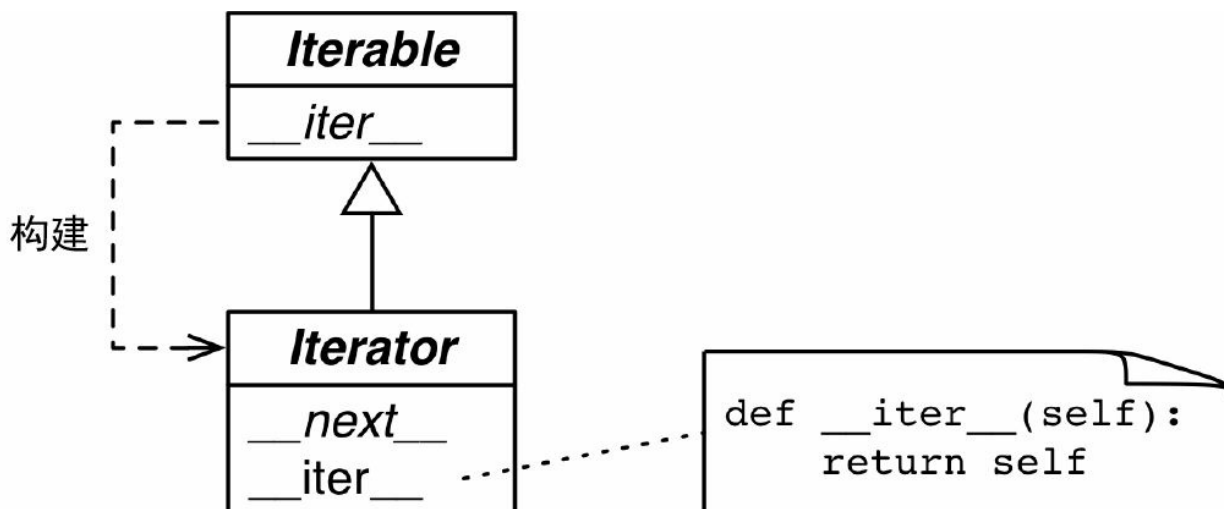
图 17-1：抽象基类 Iterable 和 Iterator。 以斜体显示的是抽象方法。具体的 Iterable.__iter__ 方法应该返回一个新的 Iterator 实例。具体的 Iterator 类必须实现 __next__ 方法。Iterator.__iter__ 方法直接返回实例本身
