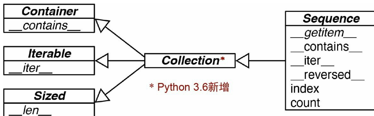
图 13-2: Sequence 抽象基类和 collections.abc 中相关抽象类的 UML 类图。箭头由子类指向超类。以斜体显示的是抽象方法。Python 3.6 之前的版本中没有 Collection 抽象基类， Sequence 是 Container 、 Iterable 和 Sized 的直接子类
