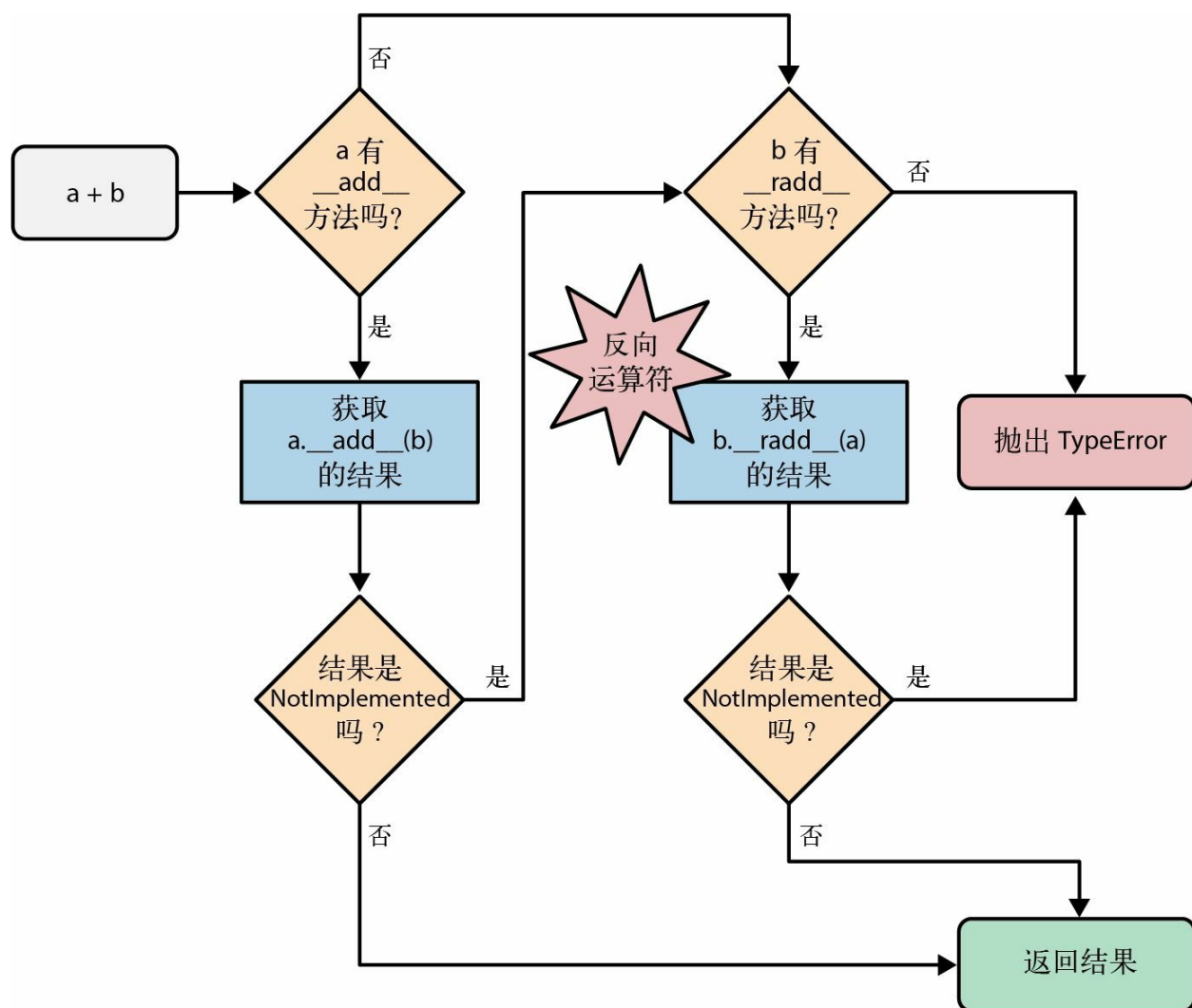
图 16-1：使用 __add__ 和 __radd__ 计算 a + b 的流程图
