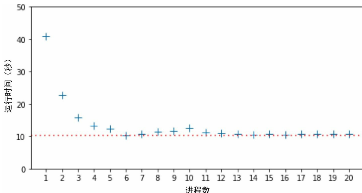
图 19-2：分别使用 1 到 20 个进程运行，得到对应的运行时间中位值。使用 1 个进程运行的中位值最大，为 40.81 秒。使用 6 个进程运行的中位值最小，为 10.39 秒（图中的虚线）
