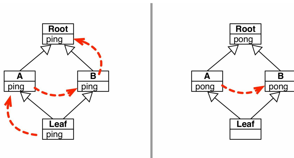
图 14-1：（左）leaf1.ping() 调用的唤醒过程； （右）leaf1.pong() 调用的唤醒过程
