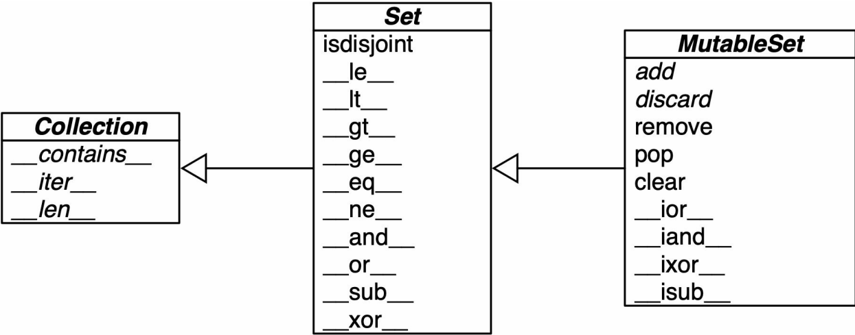
图 3-2: MutableSet 及其在 collections.abc 中的超类的简化 UML 类图（以斜体显示的名称是抽象类和抽象方法；简单起见，省略了反向运算符方法）
