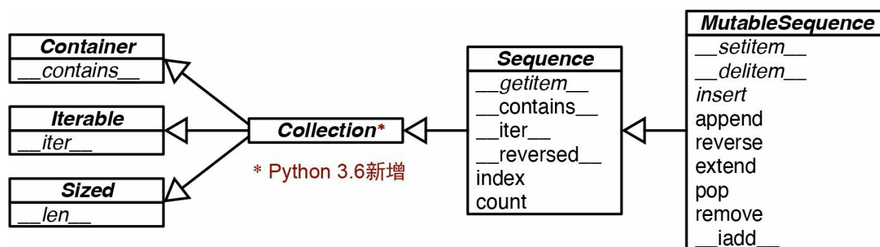
图 13-3: MutableSequence 抽象基类和 collections.abc 中它的超类的 UML 类图（箭头由子类指向祖先，以斜体显示的名称是抽象类和抽象方法）
